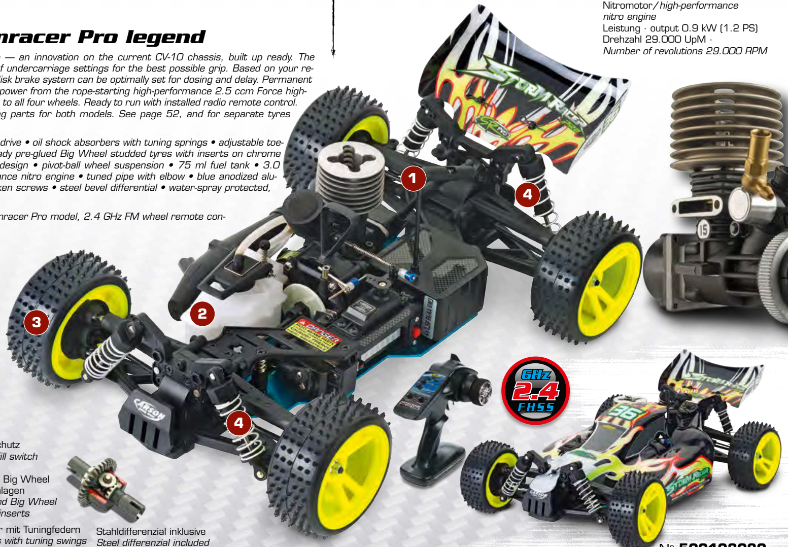
Einstellbare Scheibenbremse Adjustable disk brake
