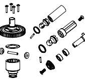
Hauptzahnrad Antriebswelle hinten Main gear rear shaft
