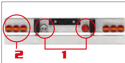
1. Nebel-/Rückfahrscheinwerfer-Set 1. Fog/backup light set N° 50 090 7077 2. 3-Kammer-Rückleuchten rund 2. 3-chamber taillights, round N° 500907039
