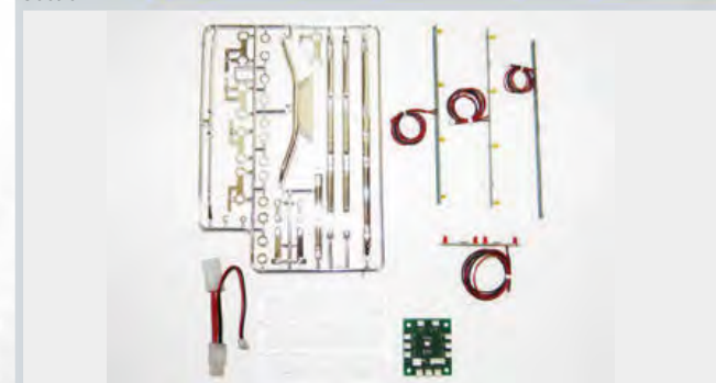
1:14 Begrenzungsleuchten mit Elektronik für 2/3-Achs EU-Zugmaschinen 1:14 Marker light with electronic fits 2/3 axle EU-Trucks. MFC kompatibel / MFC compatible
