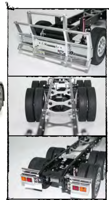
Alu Rahmenabschluss 3 Tlg. Alloy rear chassis mount N° 500530911
